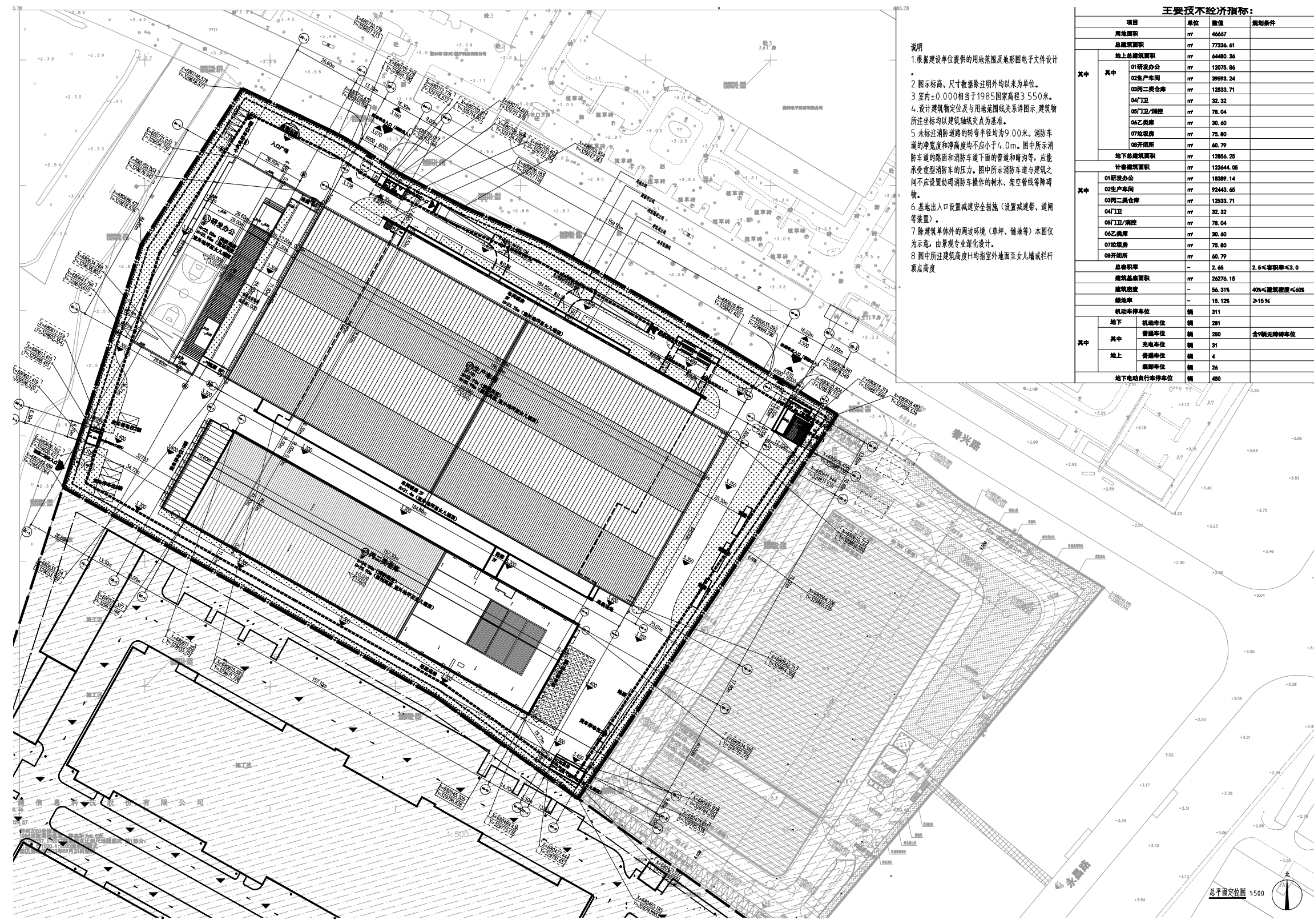
总平面图
