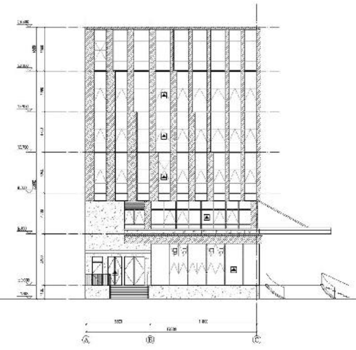
1#研发办公东立面图
