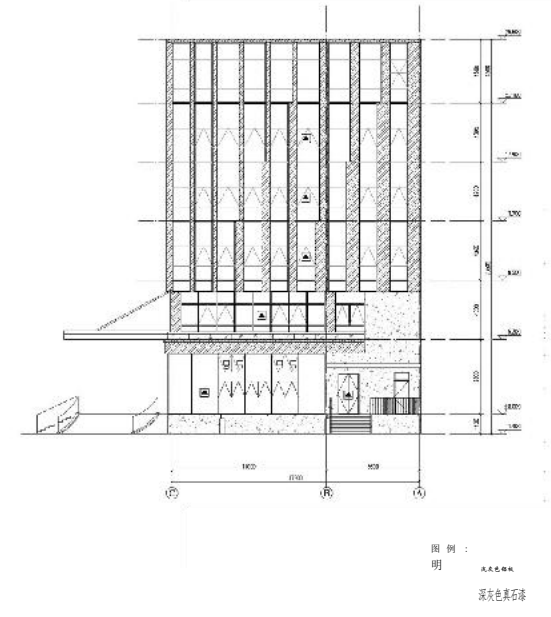
1#研发办公西立面图
