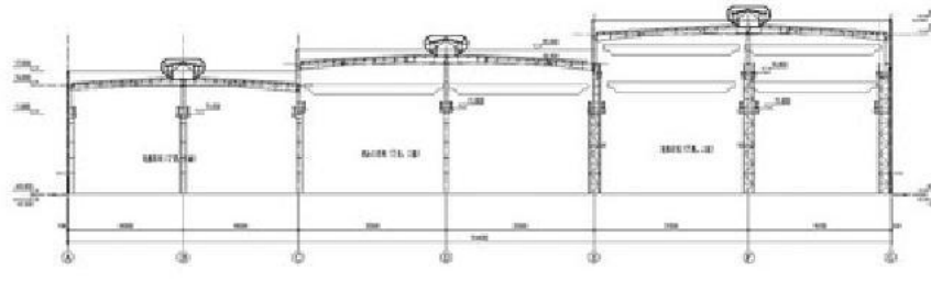
2#厂房1-1剖面图
