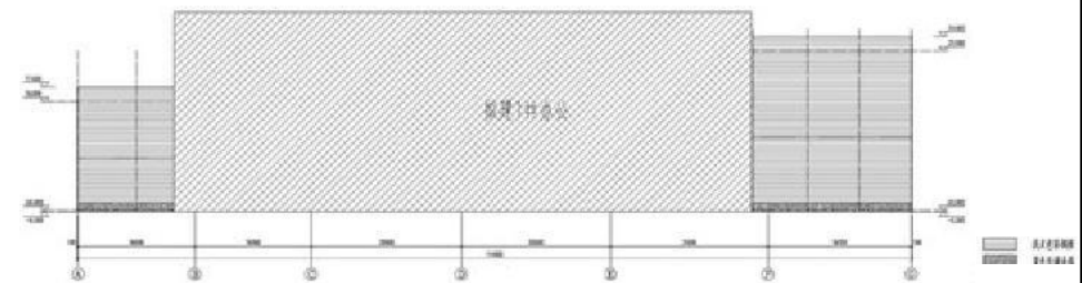
2#厂房北立面图
