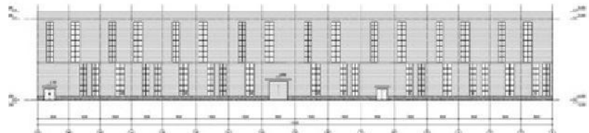
2#厂房西立面图
